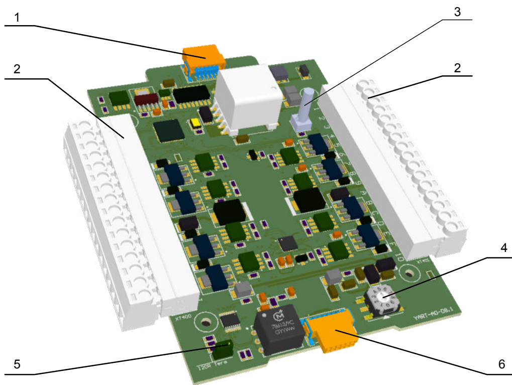
Рисунок 6 – Внешний вид платы
