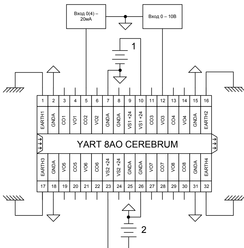
Рисунок 8. Подключение управляющих сигналов управления.
