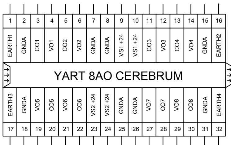
Рисунок 7 – Функциональная схема модуля расширения
