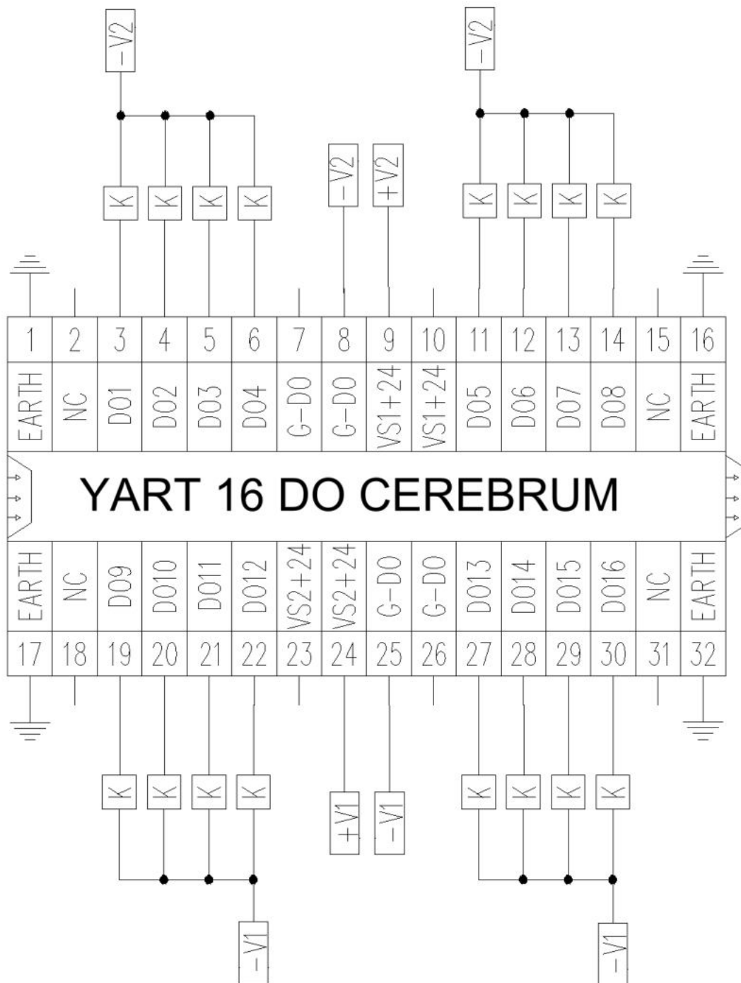
Рисунок 8. Подключение реле к выходам модуля.
