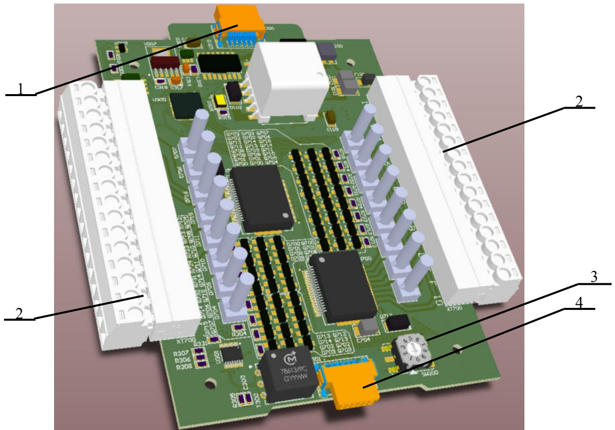
Рисунок 6 – Внешний вид платы
