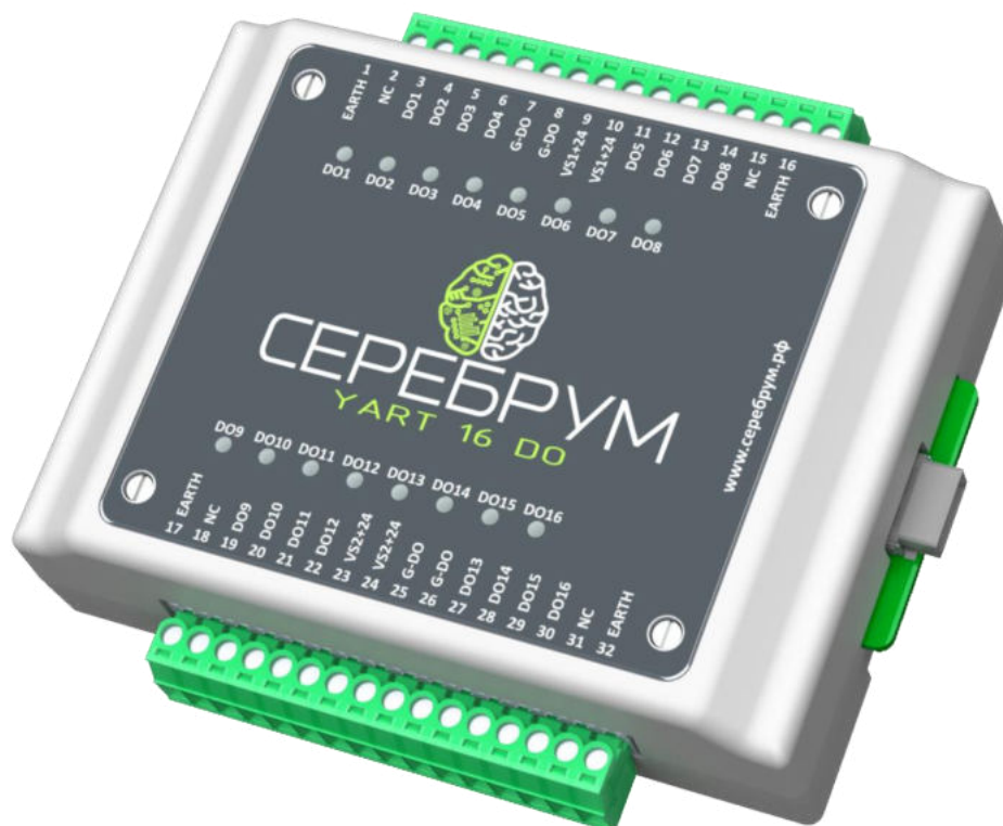
Рисунок 1 – Внешний вид модуля расширения
