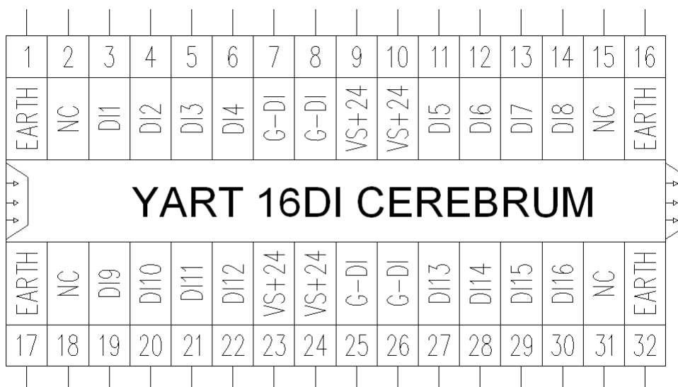
Рисунок 4 – Функциональная схема модуля расширения
