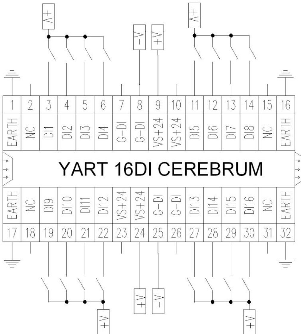
Рисунок 8. Подключение дискретных датчиков.
