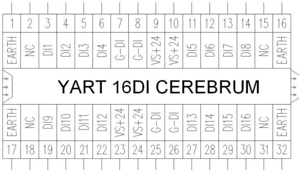
Рисунок 7 – Функциональная схема модуля расширения
