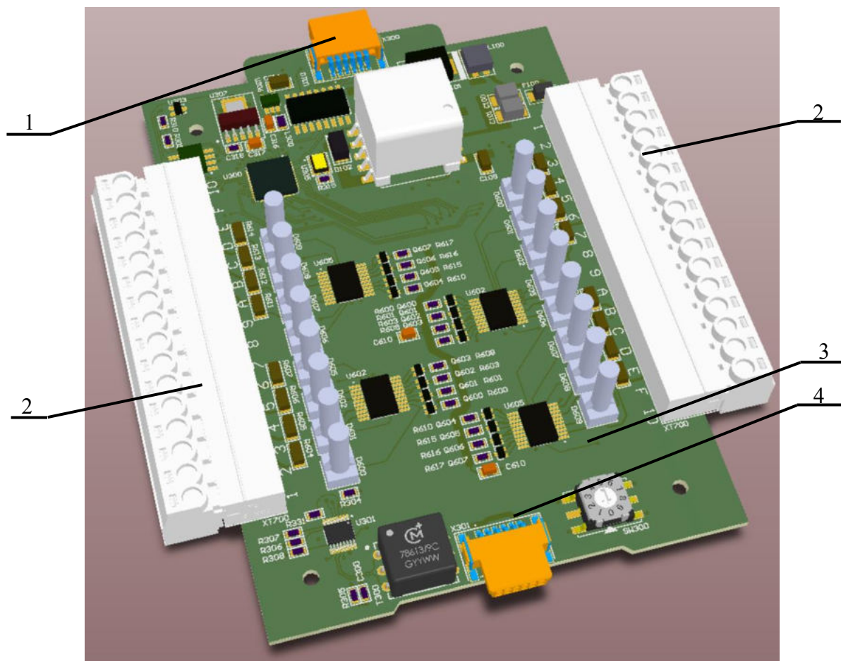
Рисунок 6– Внешний вид платы
